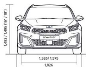
Dimensões ICE GT-Line (mm)
