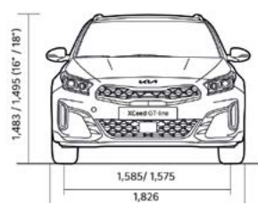
Dimensões PHEV de base (mm)
